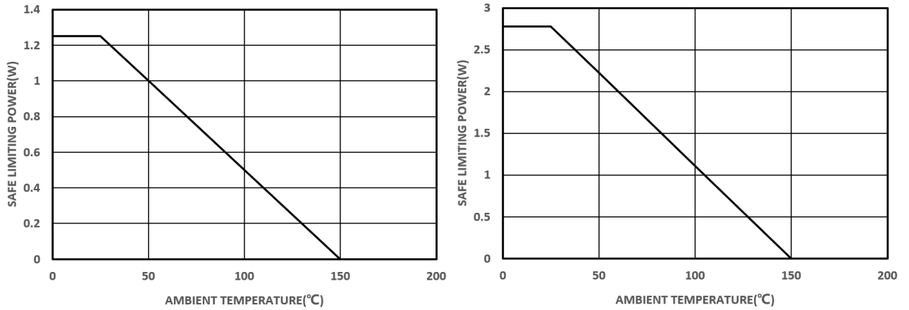
图 9. 热降额曲线, 依据 DIN V VDE V 0884-11 的安全限值与环境温度的关系(左: π12xA3x; 右: π12xA6x)
