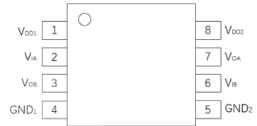
图 4. \pi 121A3x 管脚定义
