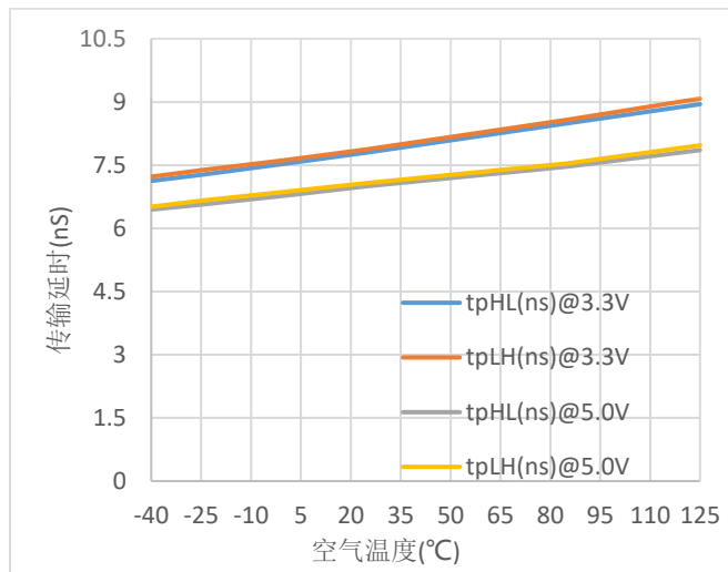
图 12. π12xA6x 传输延时 vs. 空气温度
