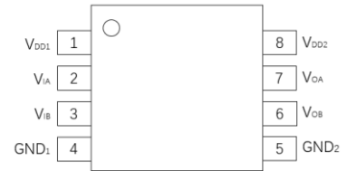
图 3. \pi 120A3x 管脚定义
