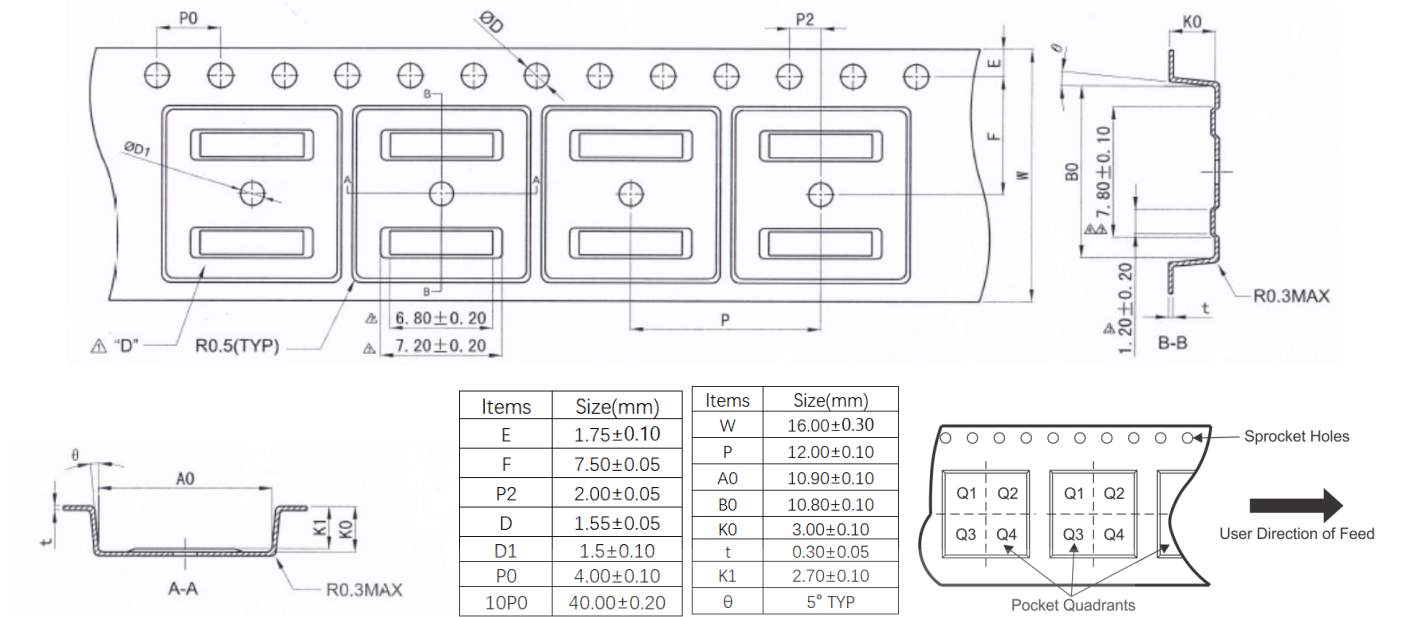
图 24.16 引脚宽体 SOIC 封装 [WB SOIC-16] 包装信息
