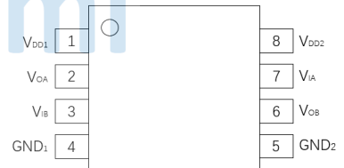
图 5. \pi 122A3x 管脚定义
