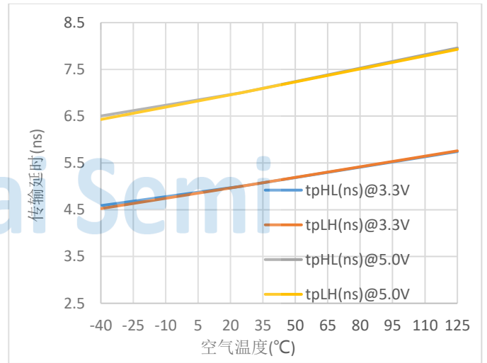
图 11. π12xA3x 传输延时 vs. 空气温度
