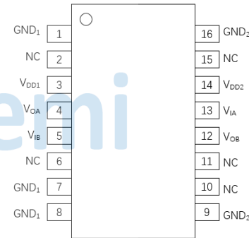
图 8. \pi 122A6x 管脚定义
