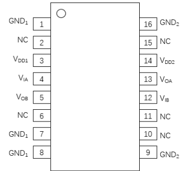
图 7. \pi 121A6x 管脚定义
