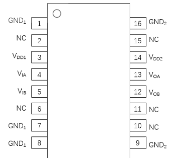
图 6. \pi 120A6x 管脚定义
