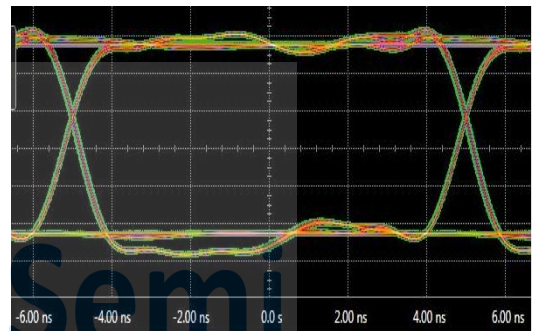
图 16. \pi 12xAxx 眼图
